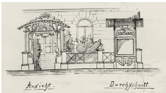
^ Saimniecības piebūves un stalla zīmējums Lielās Parka (Merķeļa) ielas pusē. 1869. gads. LNA LVVA krājums
