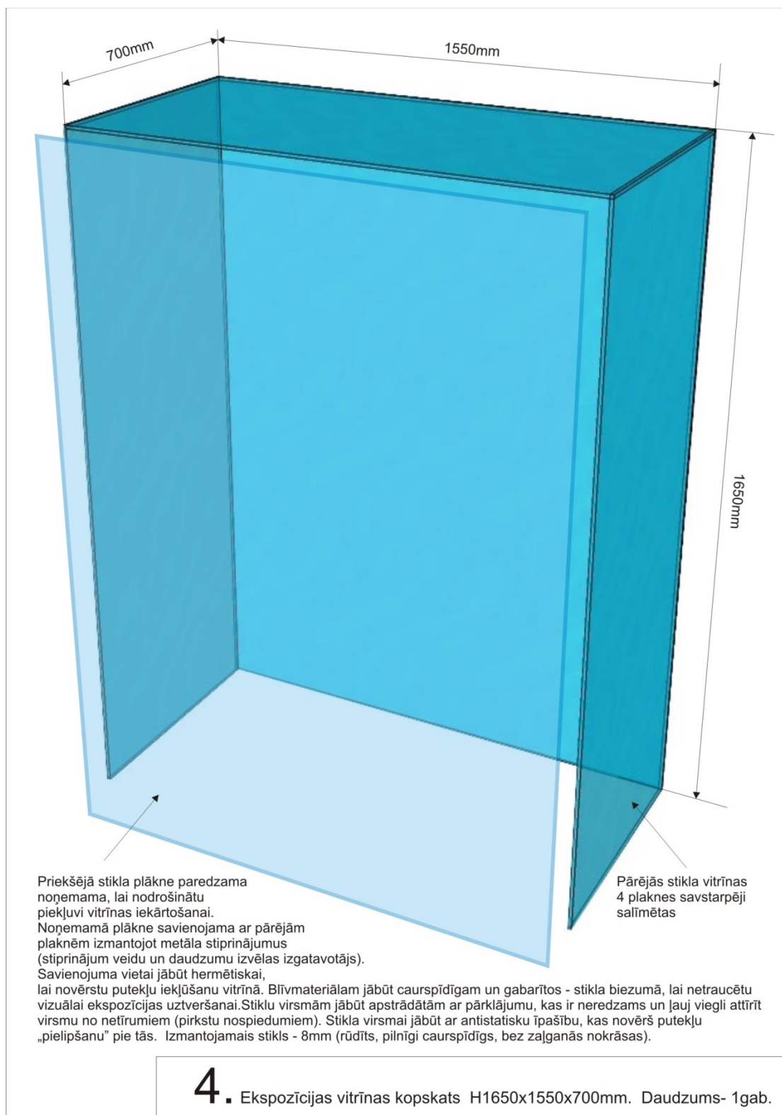
Vitrīna nr.4 – 1 gab.
