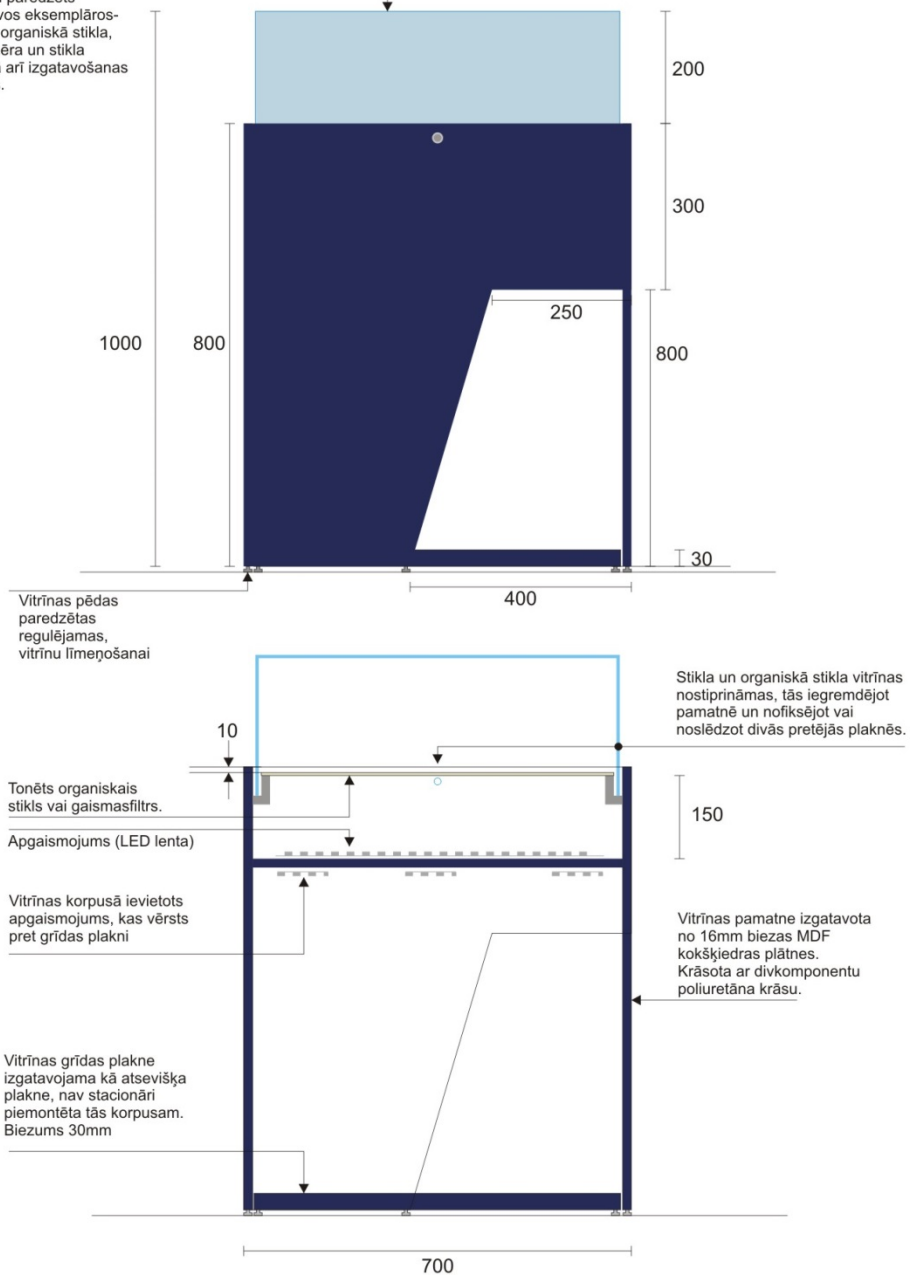
7.6. Mobīlās izstādes vitrīnas tehniskais zīmējums. Skats no mugurpuses. Mērogs 1:10. Izmēri norādīti milimetros.
