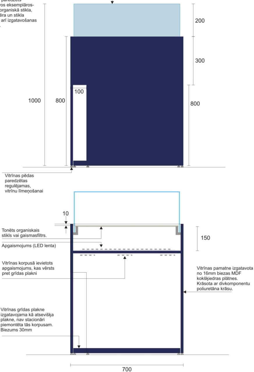
7.5. Mobīlās izstādes vitrīnas tehniskais zīmējums. Skats no kreisās puses. Mērogs 1:10. Izmēri norādīti milimetros.
