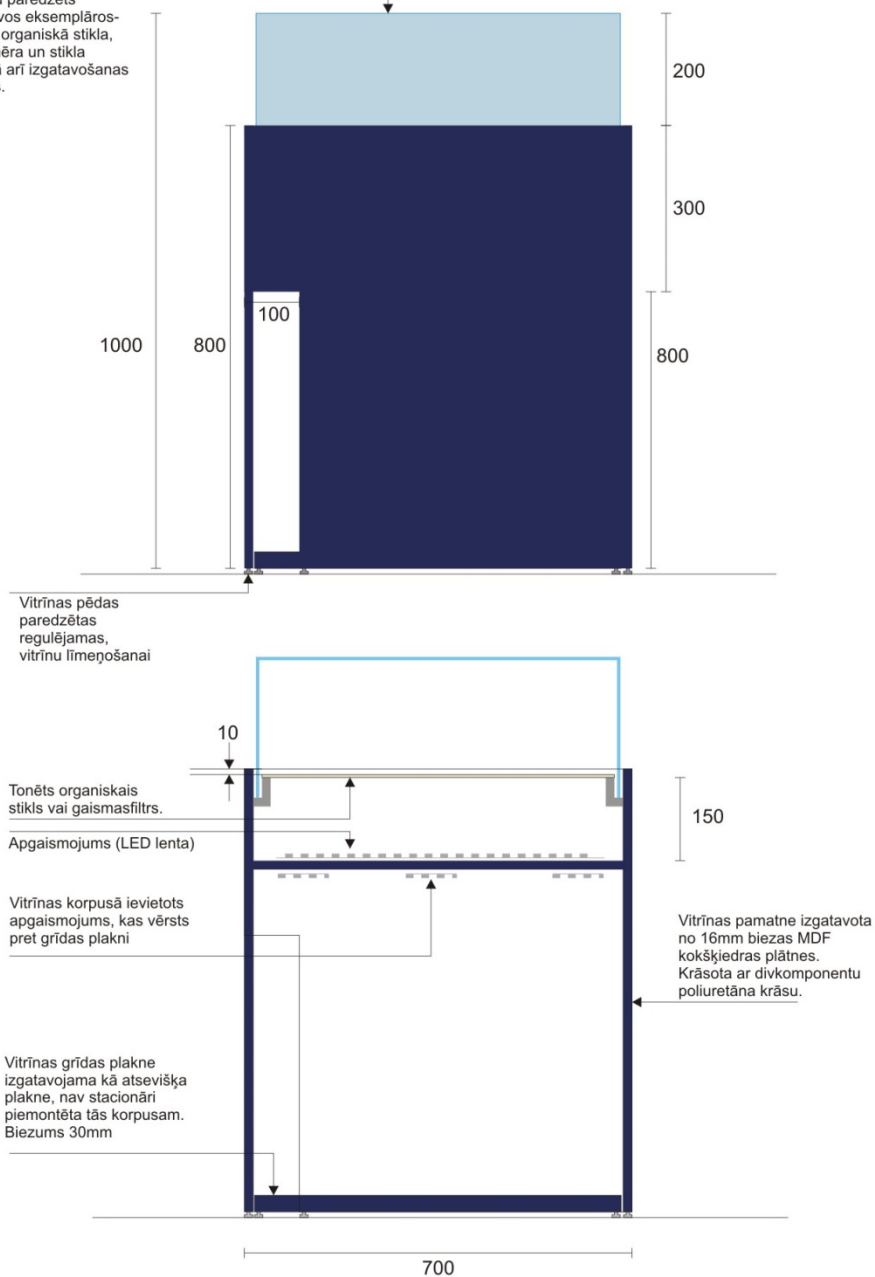
7.4. Mobīlās izstādes vitrīnas tehniskais zīmējums. Skats no labās puses. Mērogs 1:10. Izmēri norādīti milimetros.
