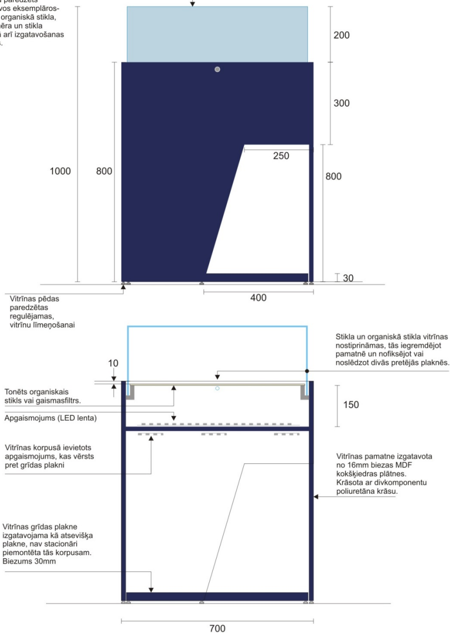
7.3. Mobīlās izstādes vitrīnas tehniskais zīmējums. Skats no priekšpuses. Mērogs 1:10. Izmēri norādīti milimetros.
