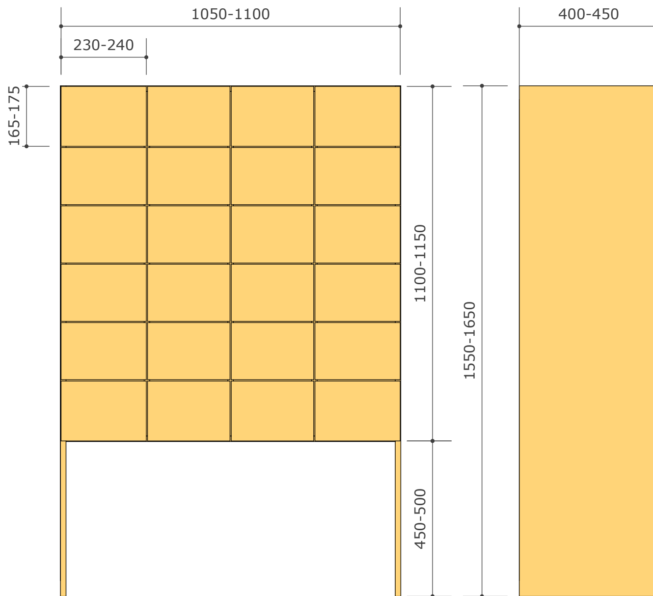
A 5 formāta kartotēkas skapis
